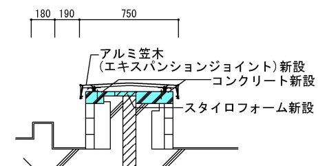
コンクリート新設後の状況
