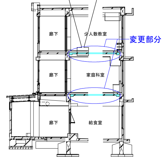
教室棟（西棟）-断面図
