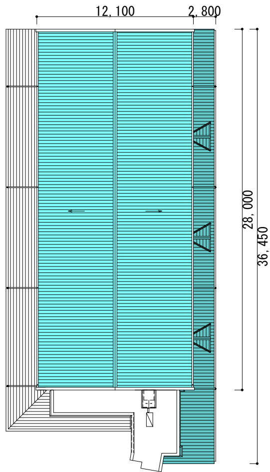
体育館棟-屋根伏図
