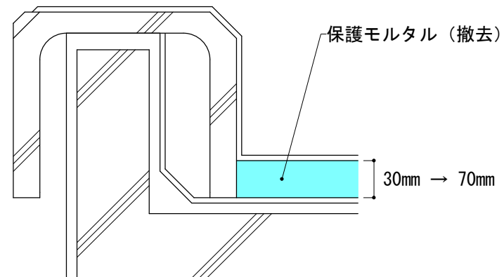
教室棟(西棟)-屋上防水層断面図
