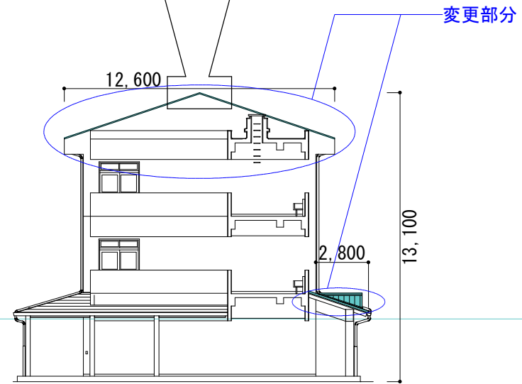
体育館棟-断面図
